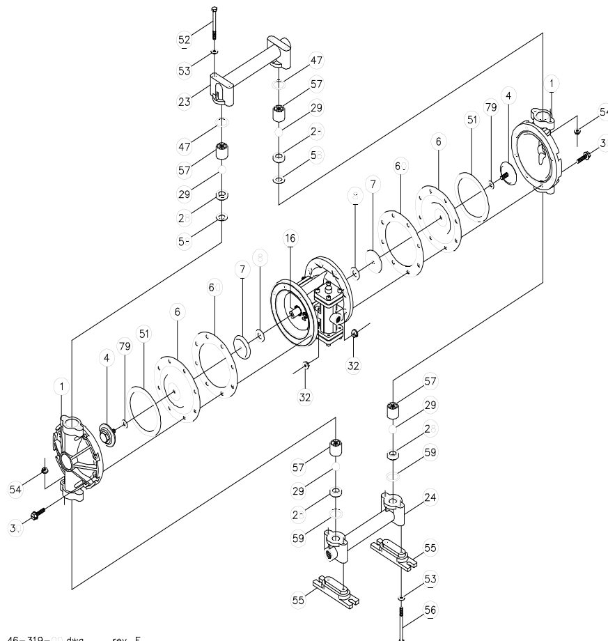
46-319-00.dwg rev. E
